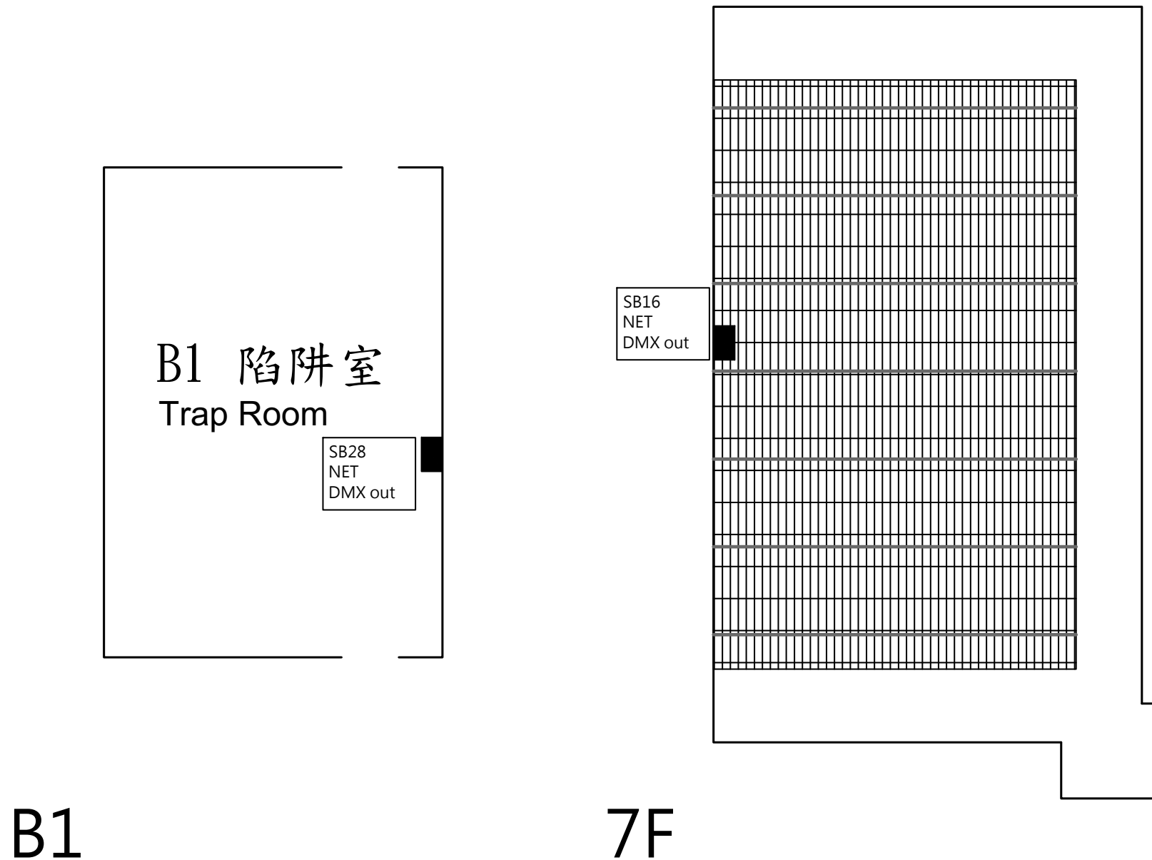
圖 ( 十七 ) 大表演廳 _ B1、7F 燈光訊號盒位置圖 Figure(17) Main Theatre _B1、7F Lighting Signal Chart
