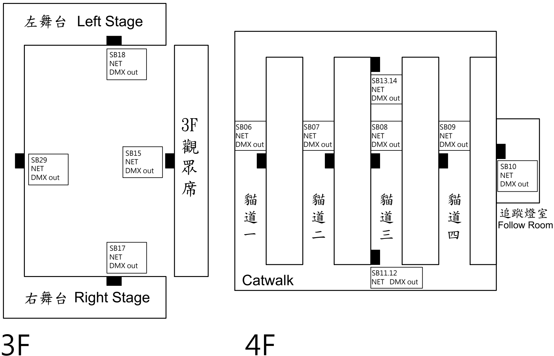
圖 (十六) 大表演廳_3F、4F 燈光訊號盒位置圖 Figure(16) Main Theatre_3F、4F Lighting Signal Chart
