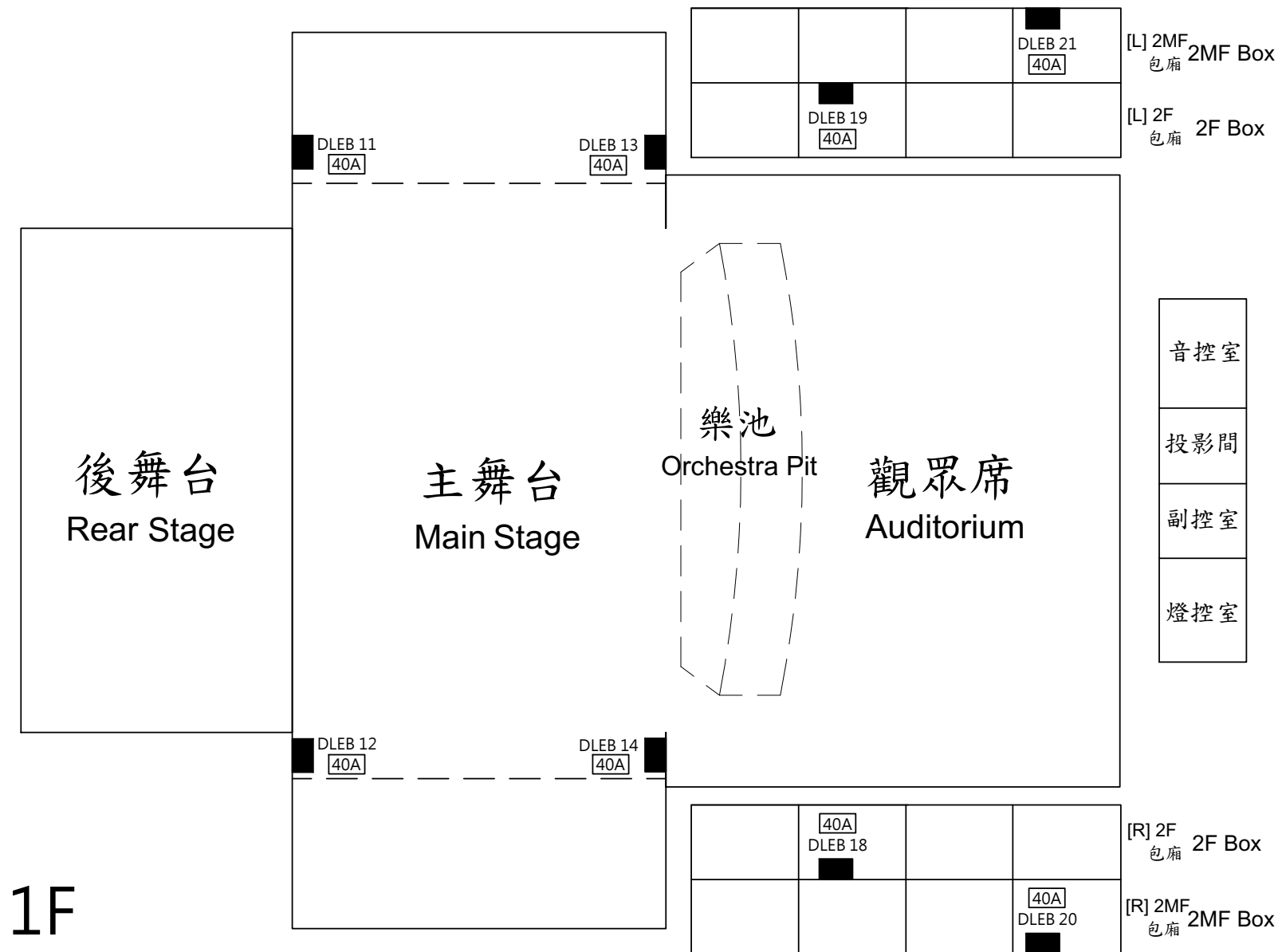
圖 (十八) 大表演廳_ 1F、2F、2MF直通電箱位置圖 Figure(18) Main Theatre_1F、2F、2MF Electricity Box
