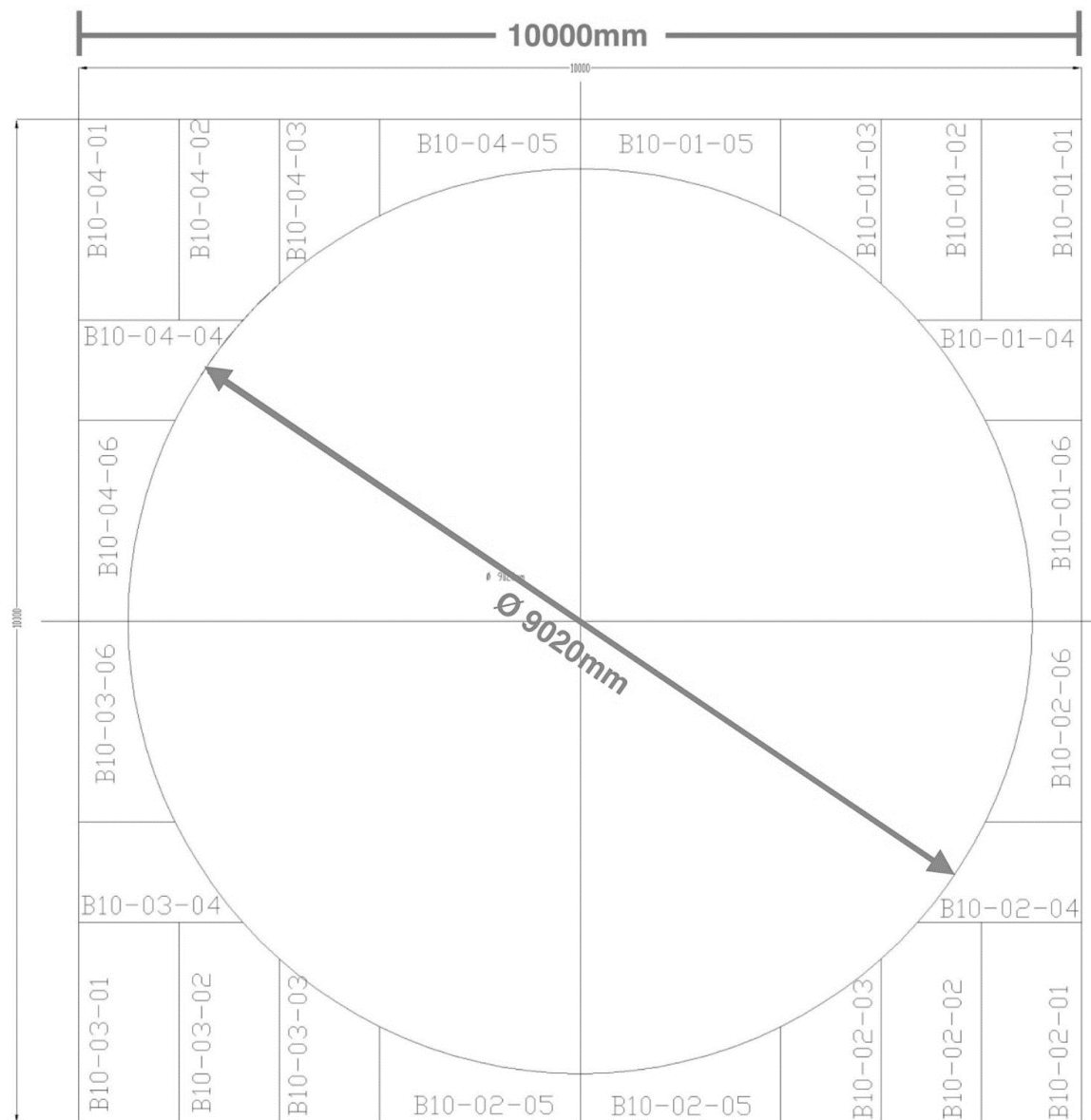
圖(六)大表演廳_旋轉舞臺10M圖示(單位:公釐) Figure(6) Main Theatre__Revolving Stage 10M Diagram (Unit: mm)
