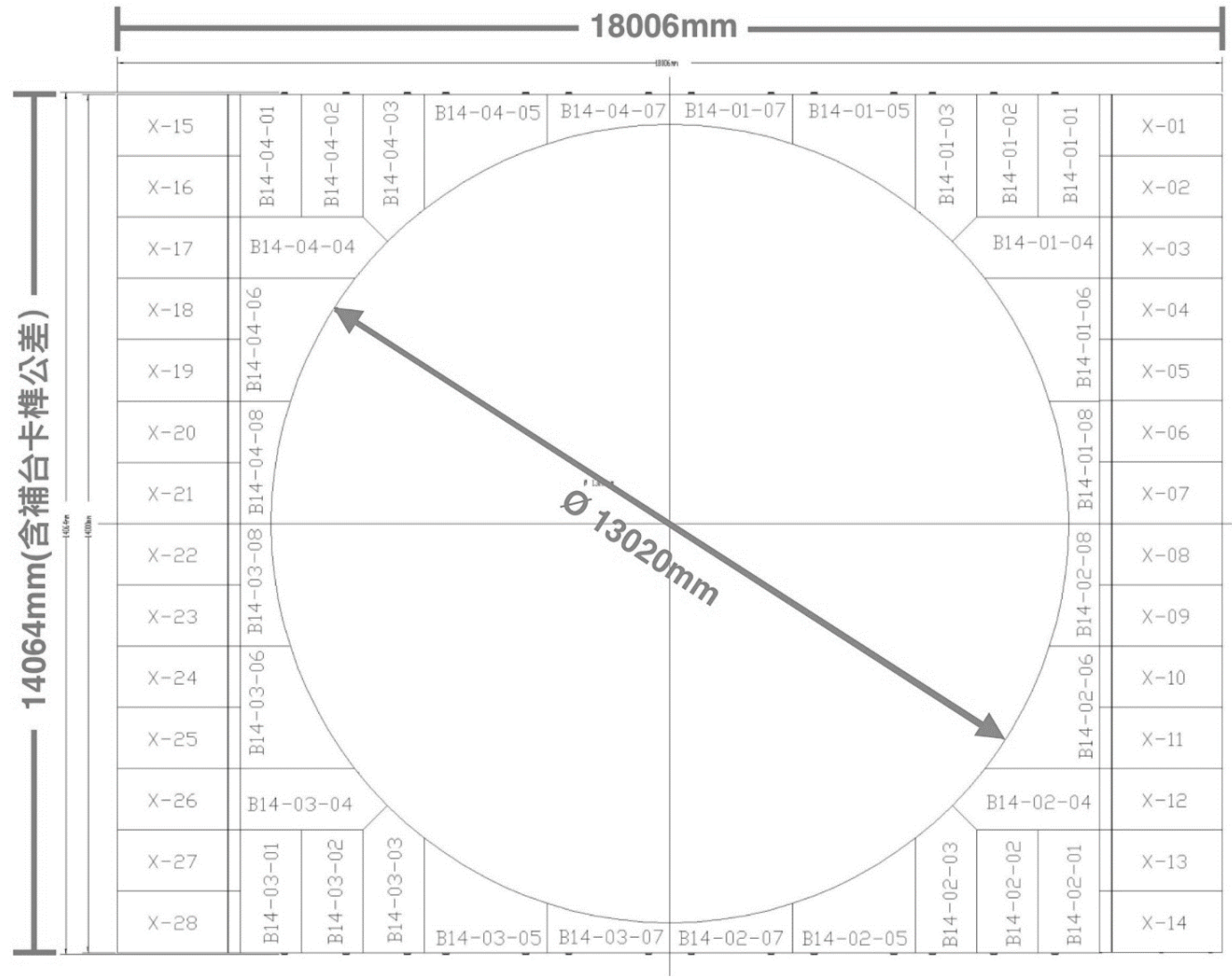
圖 ( 七 ) 大表演廳_旋轉舞臺14M圖示 ( 單位 : 公釐 )
