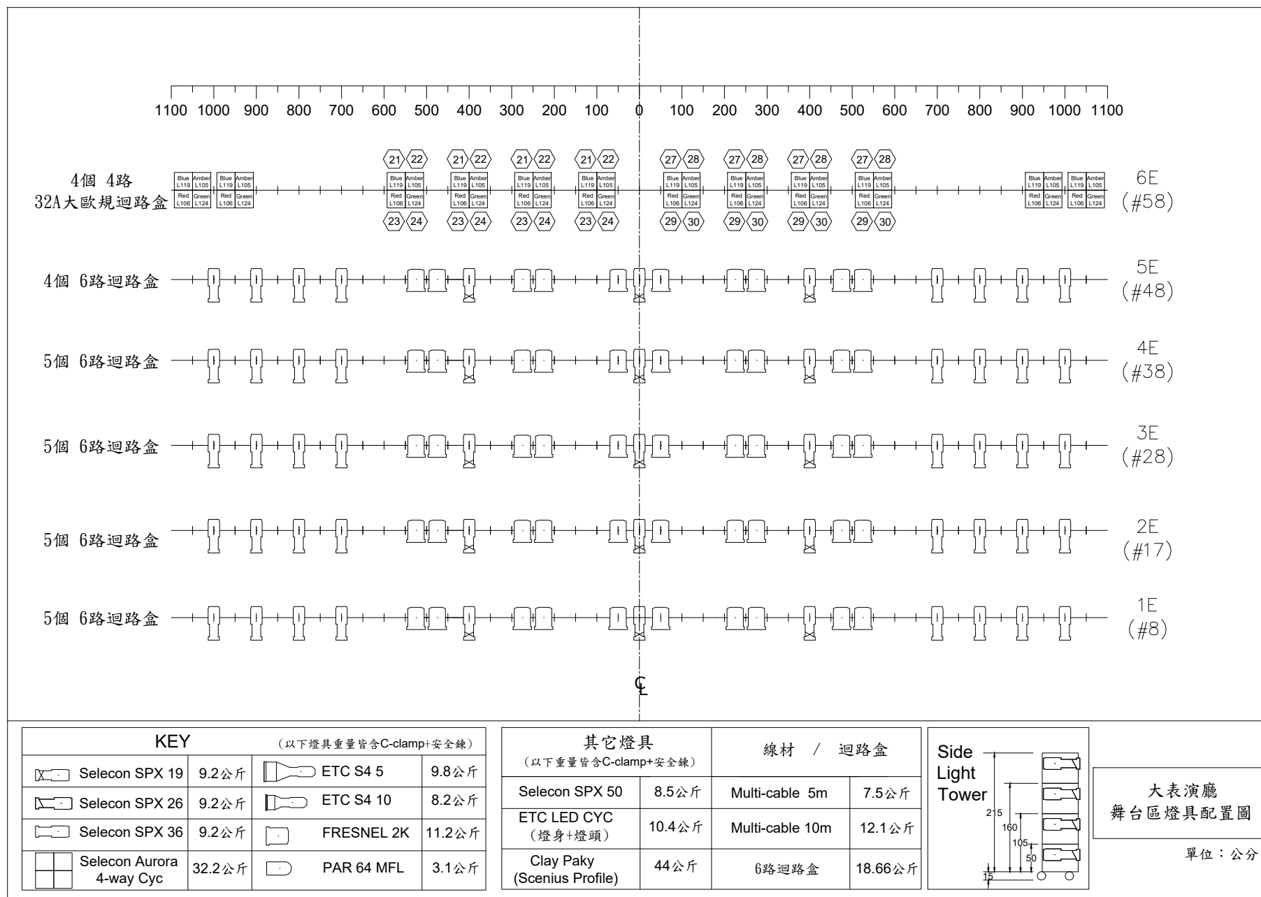
圖 (九) 大表演廳 - 舞台區_燈具配置圖 (單位：公分)
