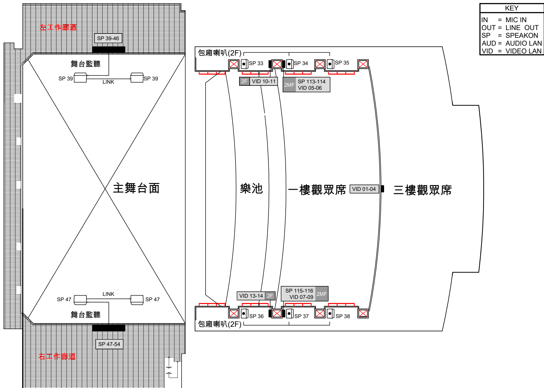
圖 (二十二) 大表演廳_ 2F、3F音響及網絡訊號迴路圖 Figure(22) Main Theatre_ 2F、3F Audio and Net Signal Chartz
