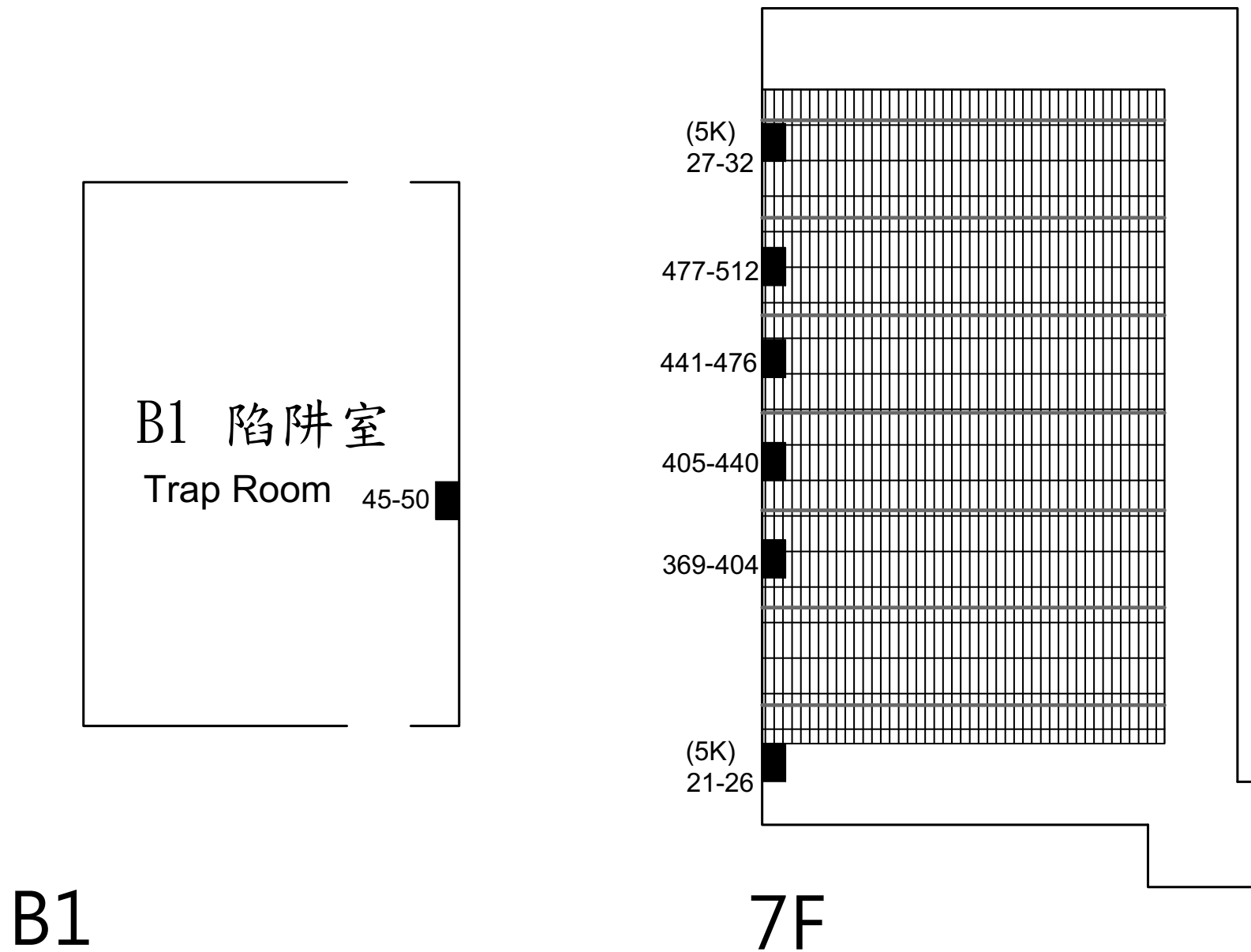
圖 (十四) 大表演廳_燈光迴路圖表 - 3 Figure(14) Main Theatre__Lighting Circuit Chart - 3
